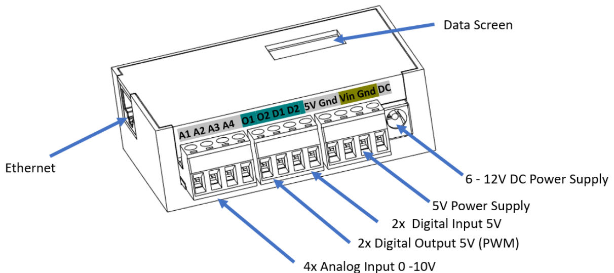
Abbildung 1 Anschluss plan ADX1-neo
